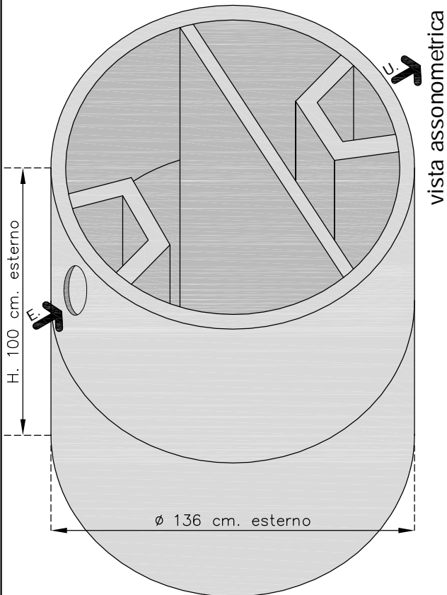
VASCA BIOLOGICA TIPO "Rovigo" DIAMETRO 125 - A 2 ELEMENTI
