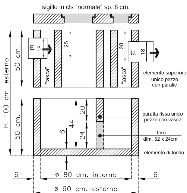
sezione A-A sc. 1:20
